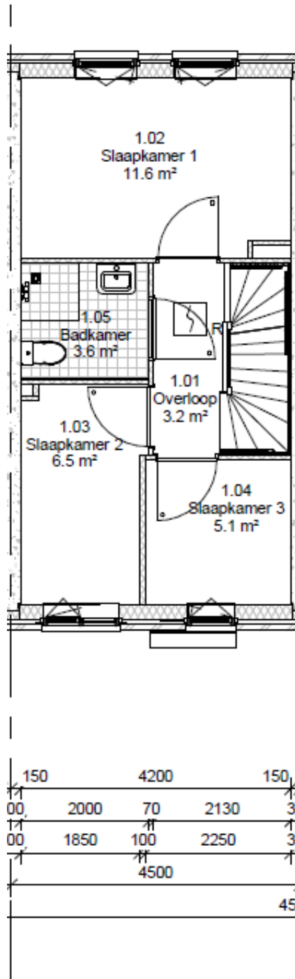
1e verdieping
