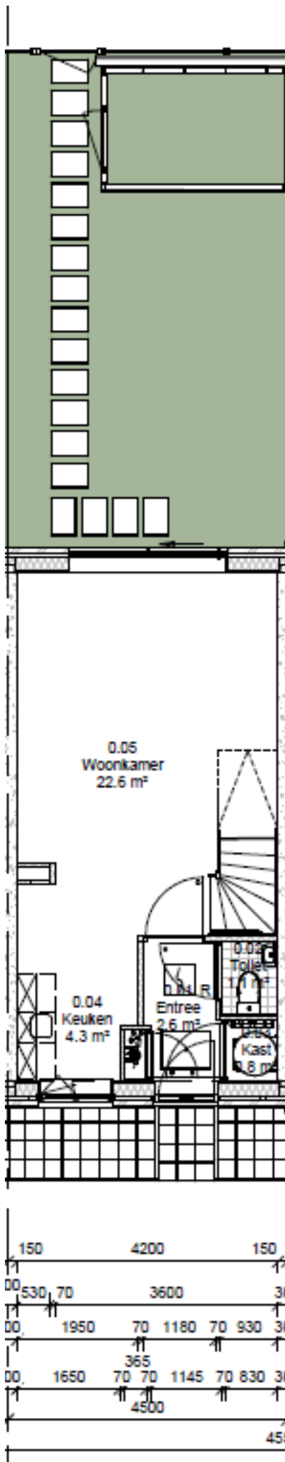
Begane grond
