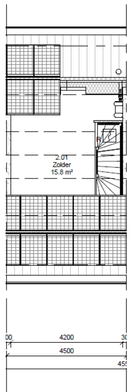
2° verdieping
